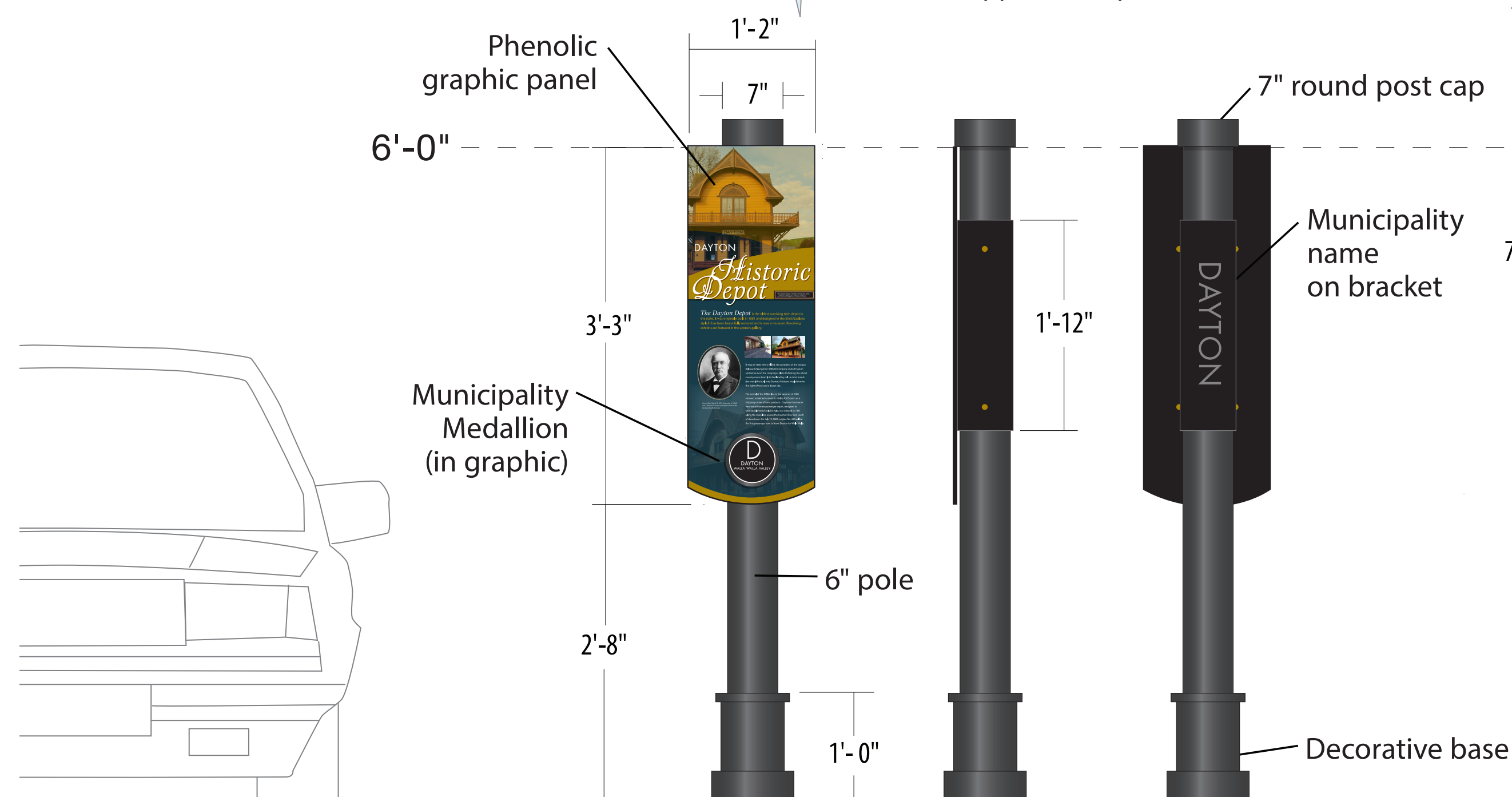
INTERP.1 Pedestrian Interpretive
