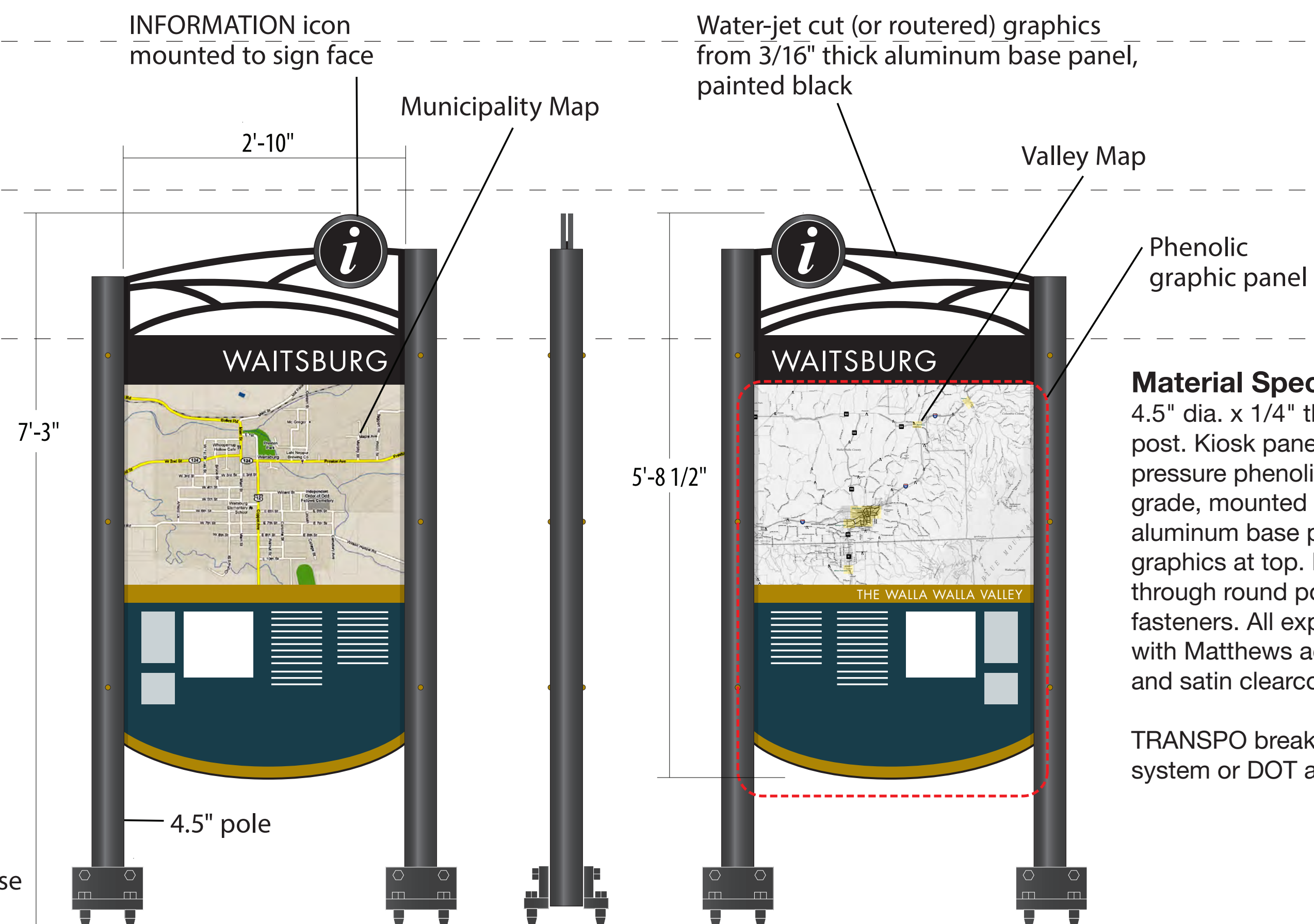
KIOSK.1 Pedestrian Kiosk (Double-sided)
